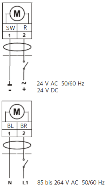
Abbildung 14: Elektrischer Anschluss M9203-Bxx
