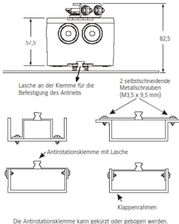
Abbildung 6: Positionierung der Antirotationsklemmen am Klappenrahmen oder Kanal
