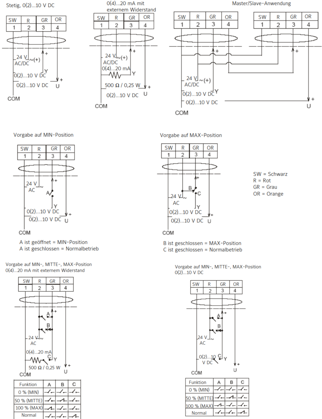
Abbildung 12: Elektrischer Anschluss M9203-GGx
