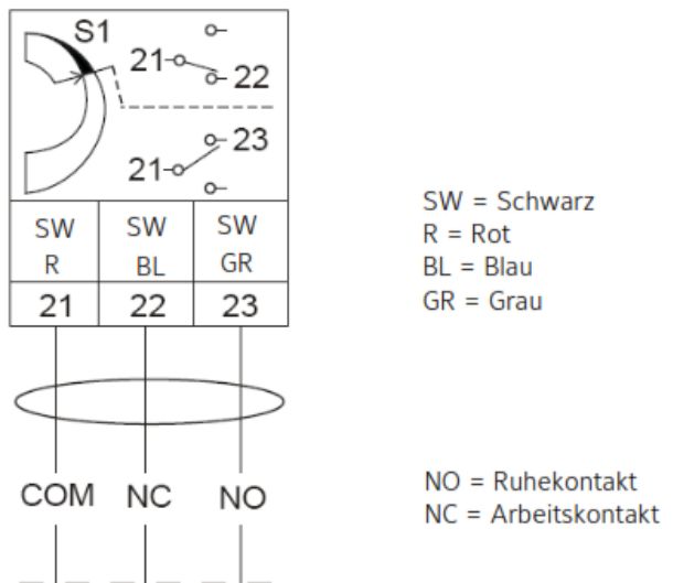
Abbildung 13: Elektrischer Anschluss M9203-AGx
