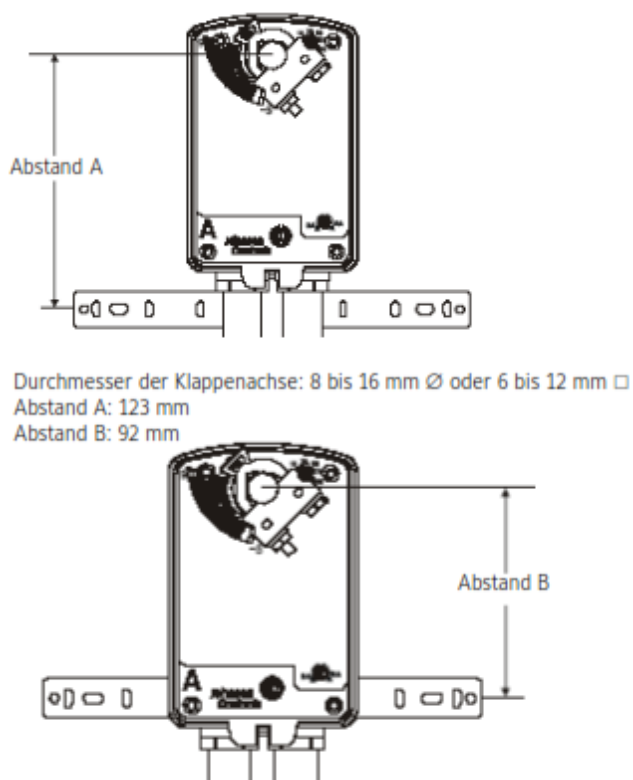
Abbildung 5: Positionierung der Antirotationsklemmen am Antrieb
