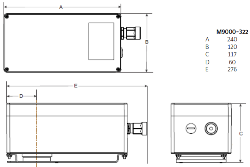
Abbildung 16: Abmessungen (mm) der Schutzgehäuse M9000-322 für M9203
