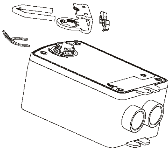
Abbildung 7: Befestigung der Kupplung
