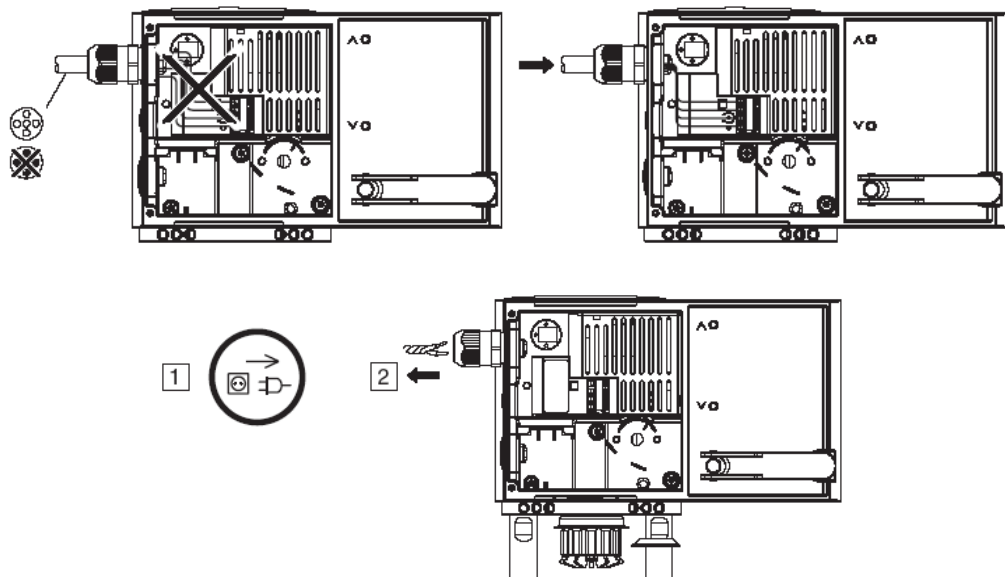
Abbildung 16: Montage von VA1000-M230N
