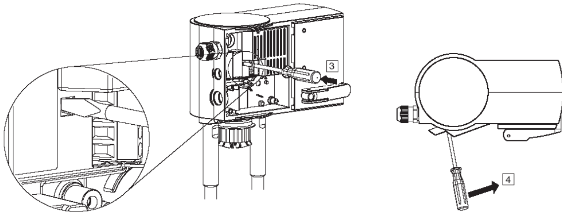
Abbildung 18: Entfernen des Moduls VA1000-M230N
