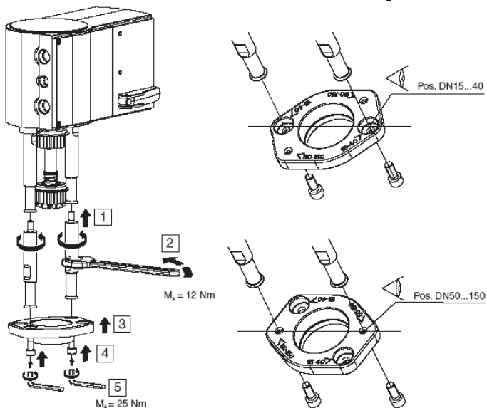
Abbildung 26: Montage VA1000-EP (Teil 1 von 3)
