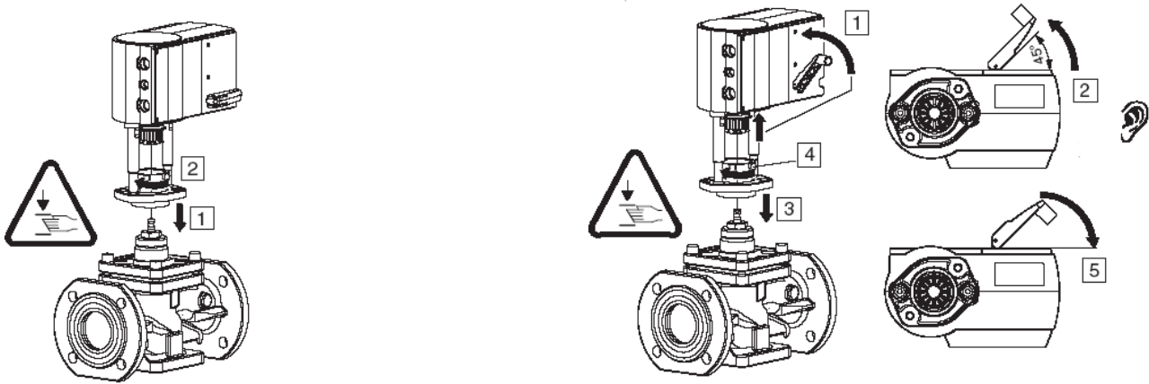
Abbildung 4: Montage der Antriebe VA1220 und VA1420
