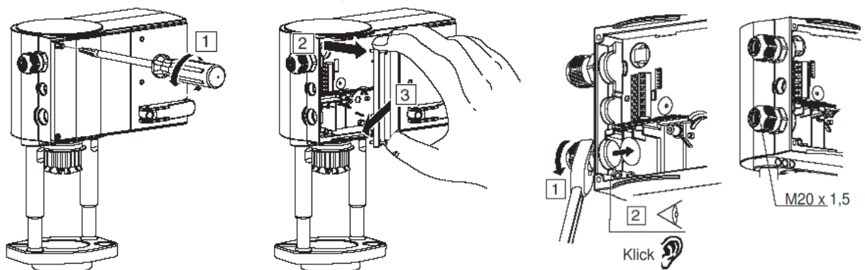
Abbildung 21: Montage VA1000-S2 (Teil 1 von 4)
