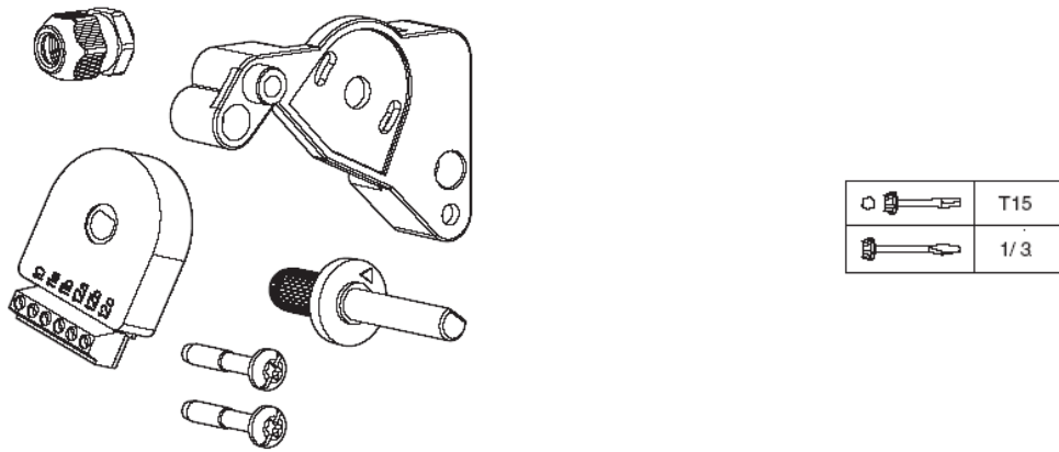
Abbildung 29: Modul Rückführpotentiometer 2 k \Omega , VA1000-P2
