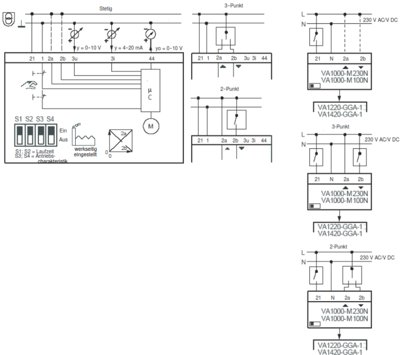
Abbildung 10: Verdrahtungsschema für VA1220-GGA-1, VA1420-GGA-1 (mit Federrücklauffunktion)
