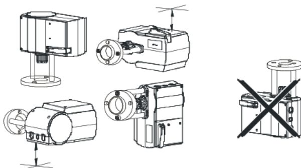
Abbildung 3: Mögliche Montagepositionen der Antriebe VA1000
