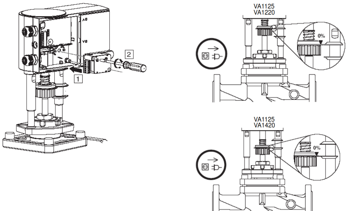
Abbildung 21: Montage VA1000-S2 (Teil 1 von 4)
