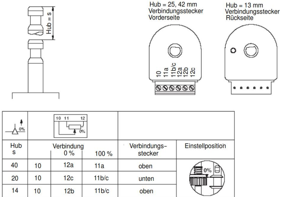
Abbildung 32: Montage VA1000-P2 (Teil 3 von 6)
