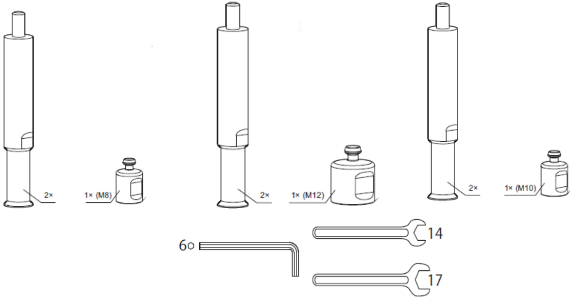
Abbildung 36: Adapterkits VA1000-ITT-KITx für PSVF, PSVD, EGSVF, EGSVD, BM
