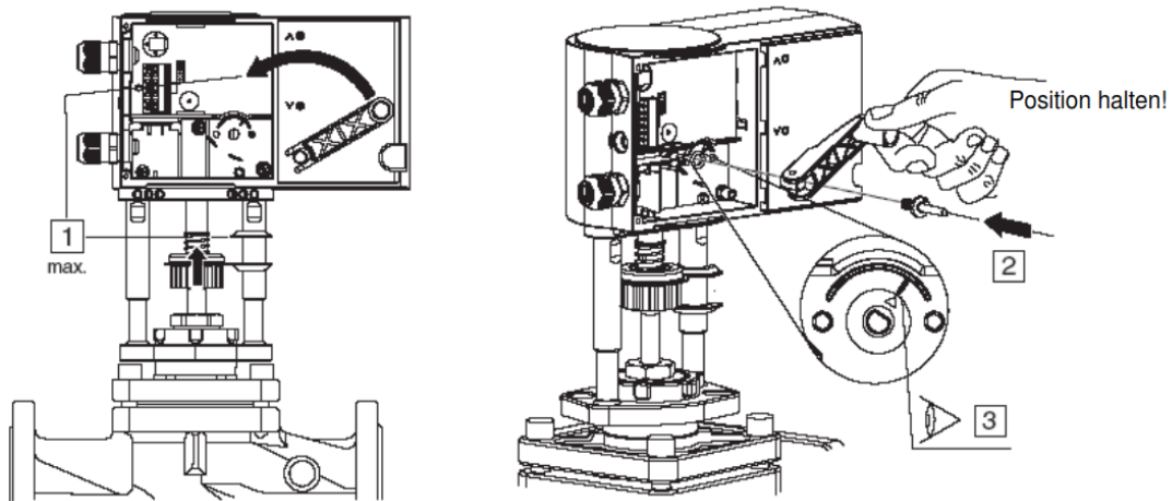
Abbildung 31: Montage VA1000-P2 (Teil 2 von 6)
