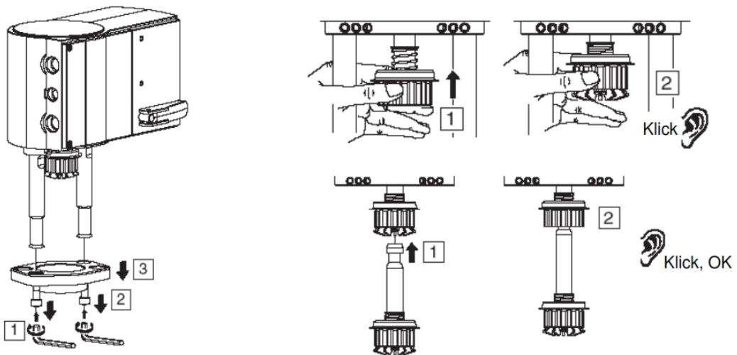
Abbildung 26: Montage VA1000-EP (Teil 1 von 3)
