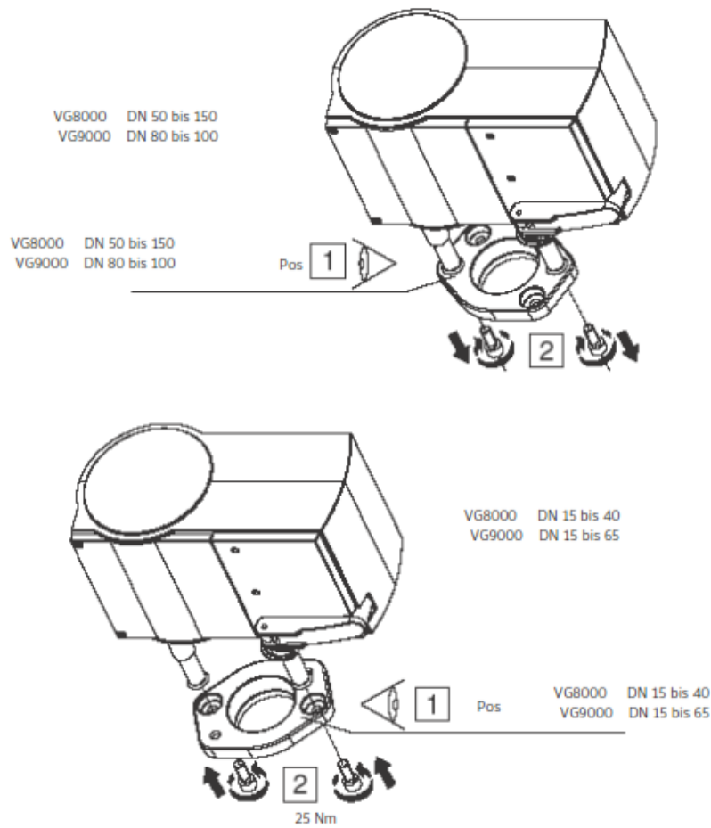
Abbildung 5: Montage des Antriebs VA1000 in Abhängigkeit von der Ventilenweite
