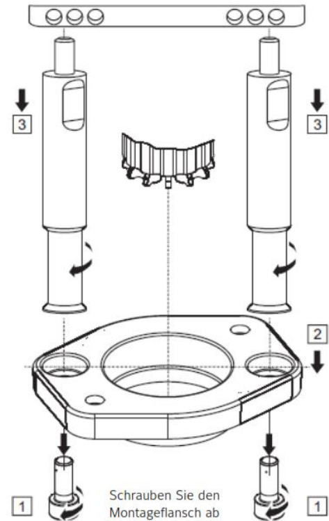
Abbildung 38: Montage des Adapterkits VA1000-ITT-KITx (Teil 2 von 3)
