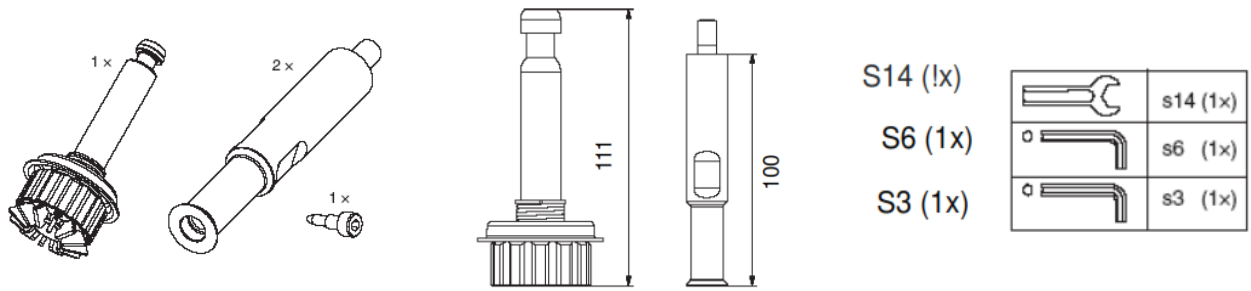
Abbildung 25: Erweiterungskit für Anwendungen von über 140 °C bis 200 °C, VA1000-EP (in mm)
