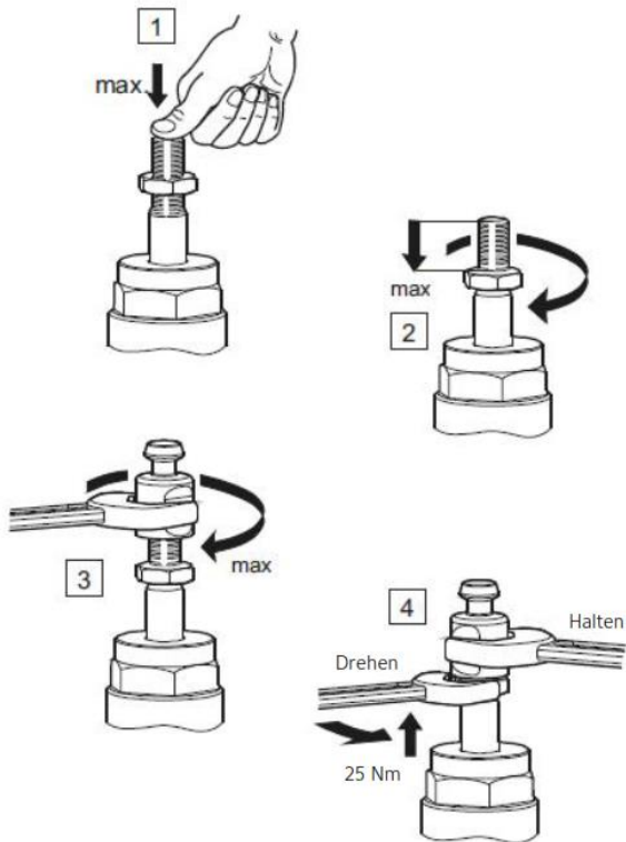
Abbildung 37: Montage des Adapterkits VA1000-ITT-KITx (Teil 1 von 3)
