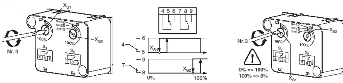
Abbildung 23: Montage und Verdrahtung VA1000-S2 (Teil 3 von 4)
