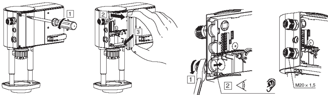
Abbildung 30: Montage VA1000-P2 (Teil 1 von 6)
