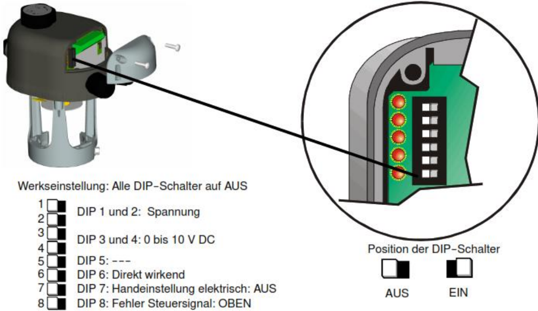
Abbildung 9: Einstellen von Wirksinn, Hub und Aufteilung des Stellbereichs an der Kabeleinheit
