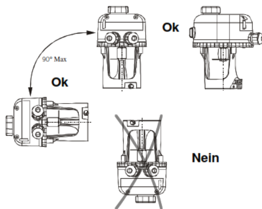
Abbildung 2: Montage des Antriebs VA-77xx
