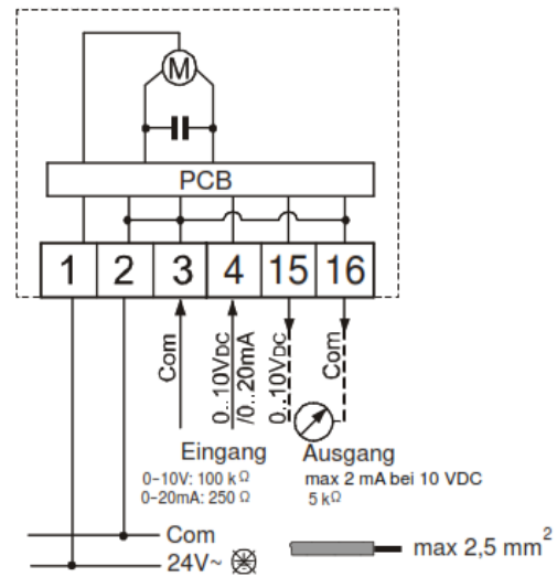
Abbildung 8: Elektrischer Anschluss VA-7746-xx01 (stetig, 24 V AC ohne Handeinstellung)
