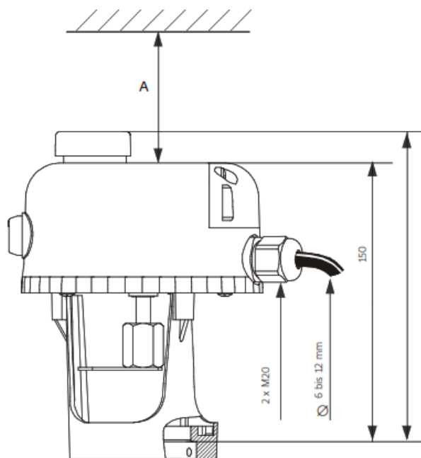
Abbildung 1: Abmessungen (mm) Antrieb VA-77xx
