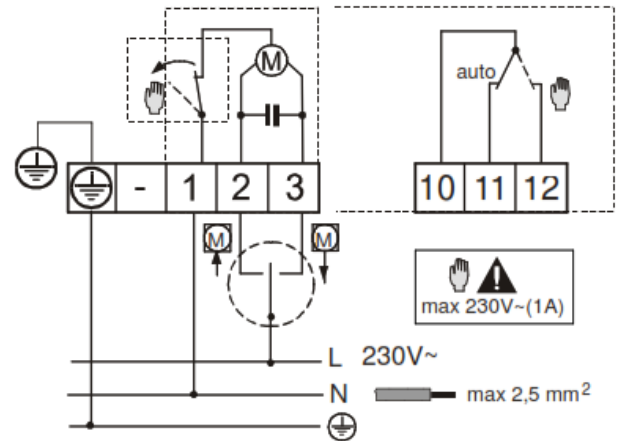
Abbildung 4: Elektrischer Anschluss VA-7740-xx03 (3-Punkt-Ansteuerung, 230 V Handeinstellung mechanisch)
