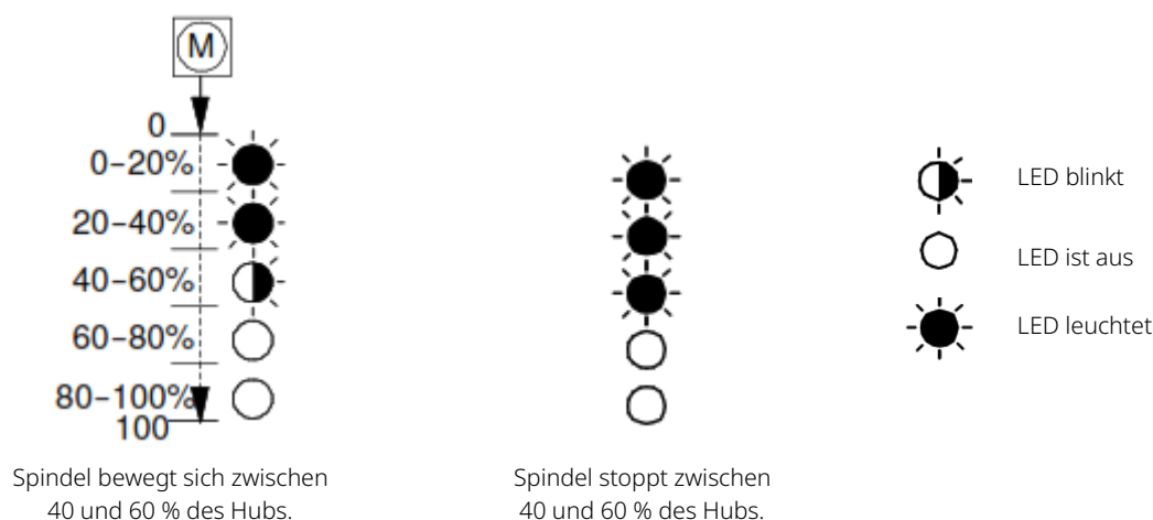
Abbildung 13: Position der Spindel wird durch die LEDs angezeigt (nur beim stetigen Antrieb VA-77x6)
